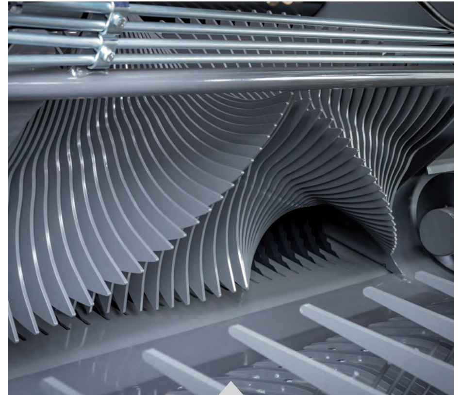
Der Rotor Xtracut 25 im spiralförmigen 4-Blatt-Design liefert eine extreme Schnittleistung
