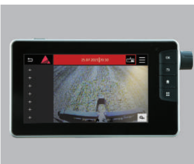
Na lis s připravenou kabeláží lze snadno přidat videokameru. Terminál balíčky FieldStar 5 zobrazuje plně barevné video a je kompatibilní v základní výbavě.
