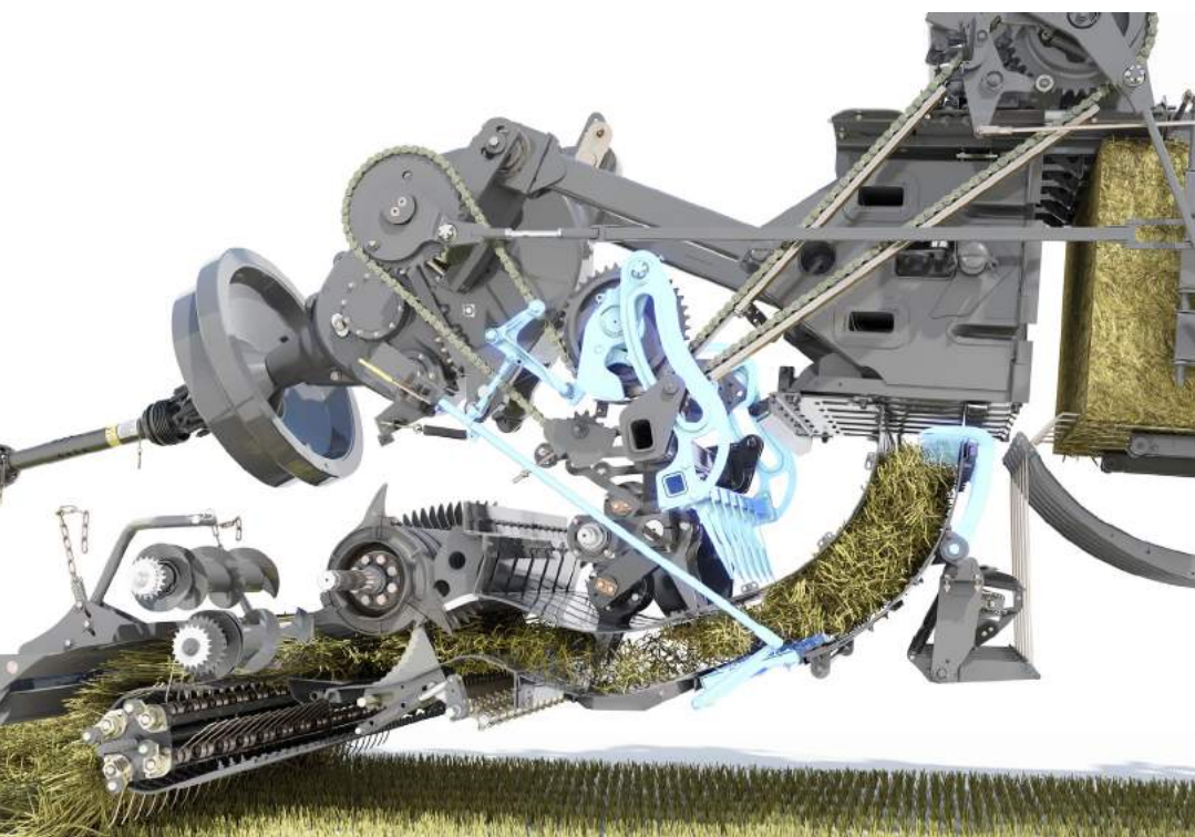
Předlisovací komora – plnění.
