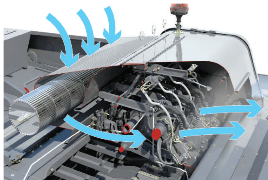
Ventilátor uzlovače
