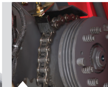
Automatické promazávání řetězu po celé šířce řetězu.
